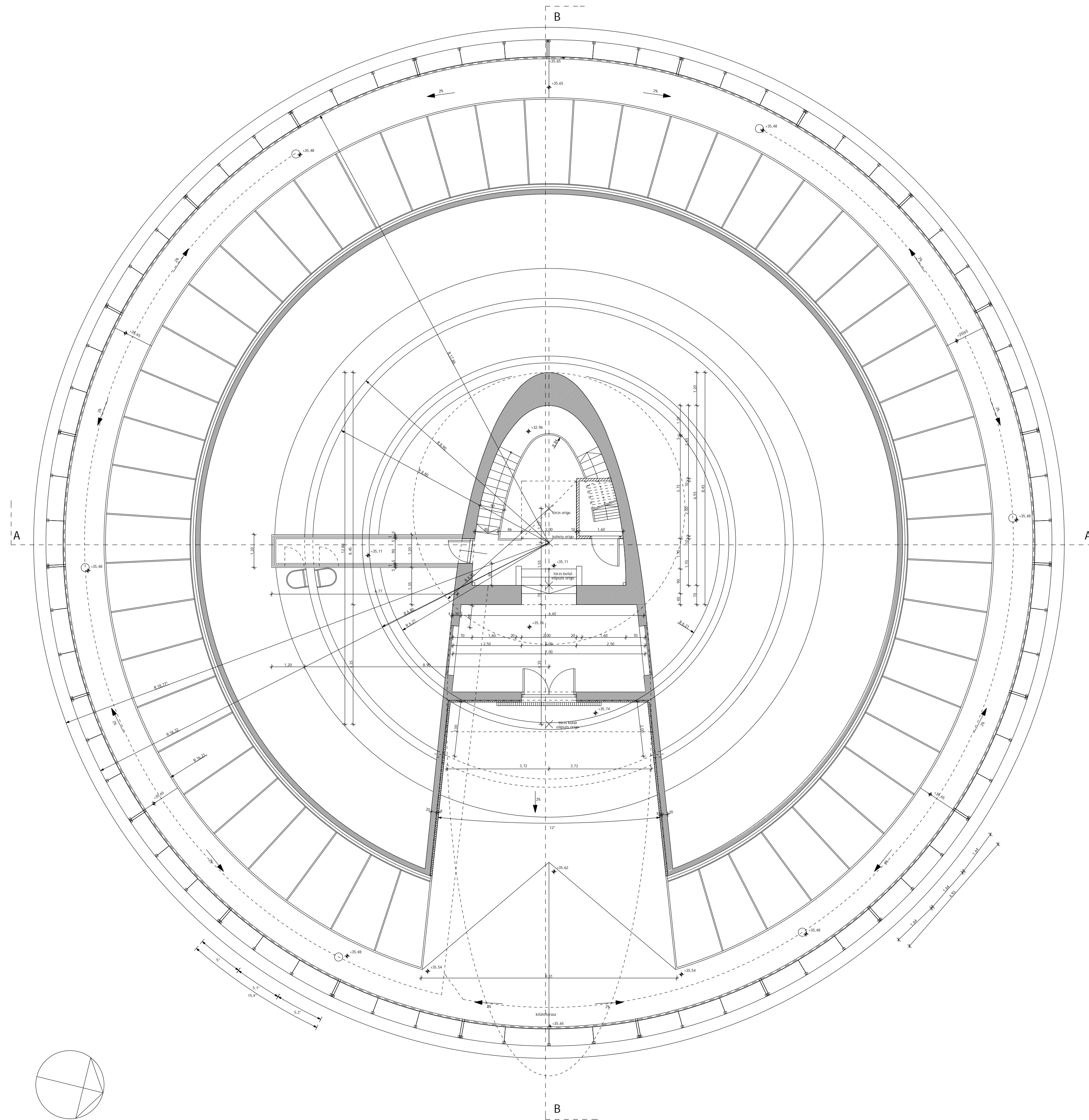
kilátó terasz szintjén alaprajz
